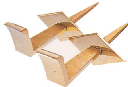
菱座額受金具 1組(打込式)
